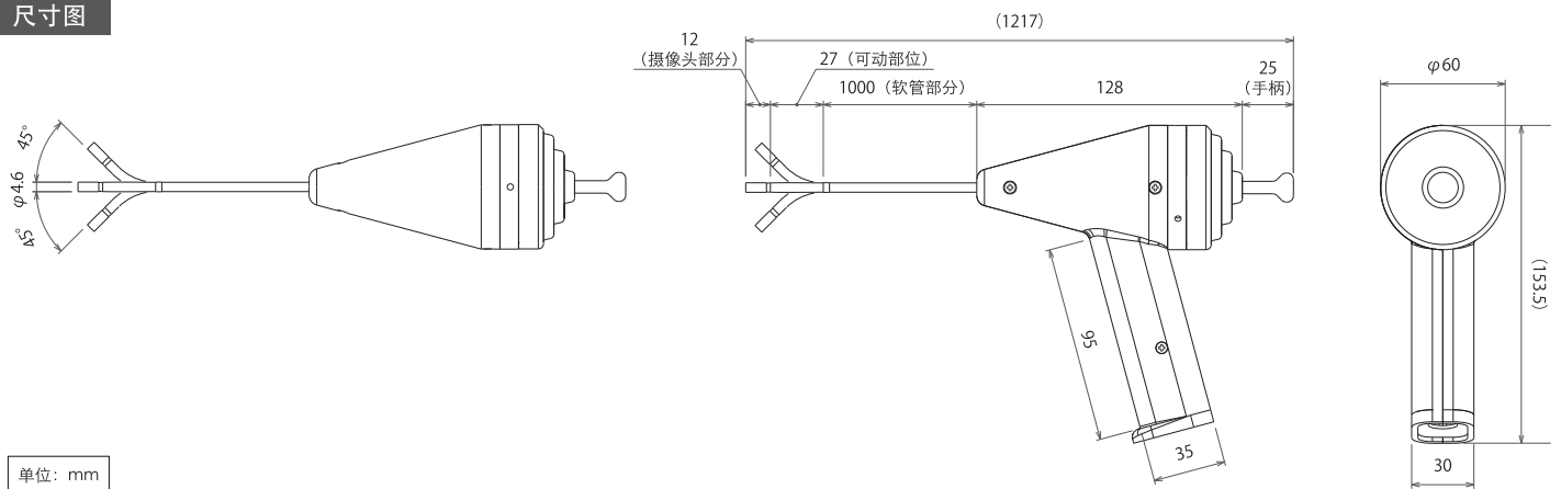
极细端部可动型工业用内视镜配置一览
